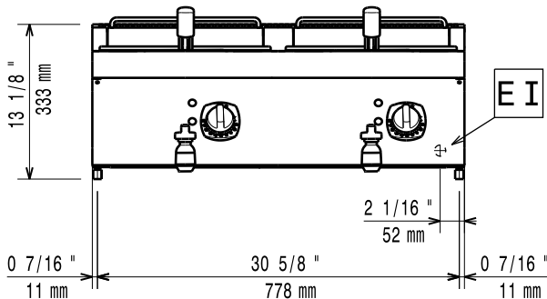
Front aanzicht
