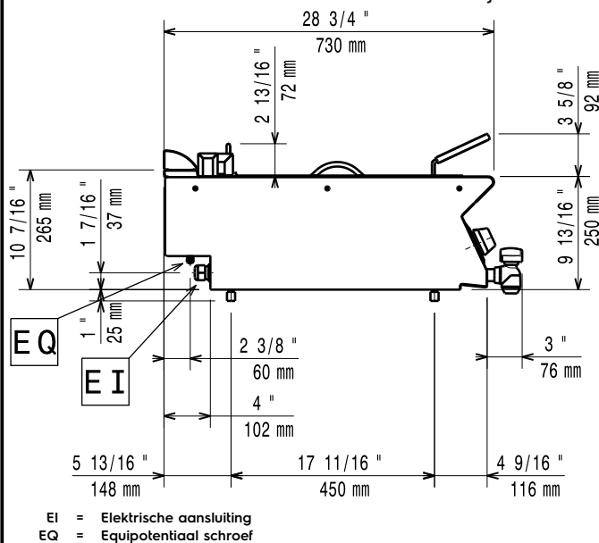
Zij aanzicht
